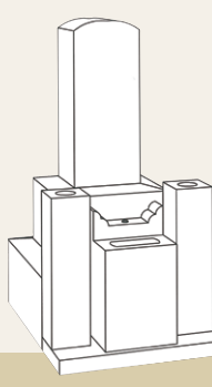
夫婦墓(前置付)
