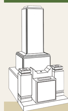
三重型二重台 (銀杏面彫り)
